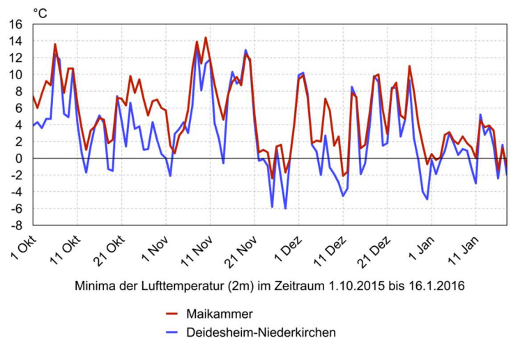
Abb. 2: Tägliche Tiefsttemperaturen an den benachbarten Klimastationen Maikammer und Deidesheim-Niederkirchen vom 01.10.2015 bis 16.01.2016
