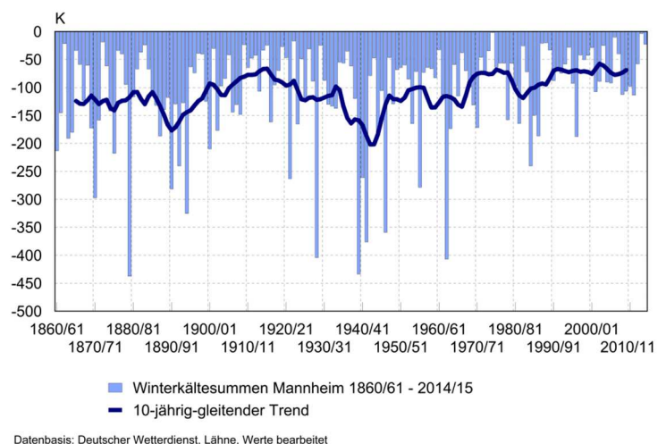
Abb. 3: Winterkältesummen an der Wetterstation Mannheim 1860/61 bis 2014/15 (K = Grad Kelvin)
