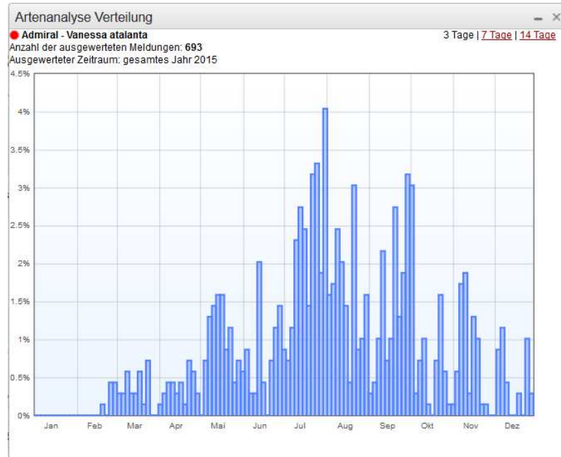
Abb. 4: Admiral - Meldezeit-Diagramm für das Jahr 2015. 49 Meldungen im November und 28 Meldungen im Dezember. Quelle: ArtenFinder/ArtenAnalyse
